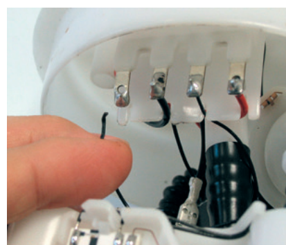
Fig. 3: Imagem de danos típica: o cabo do sensor do depósito está solto e as lâminas de contato elétrica estão empenadas.
